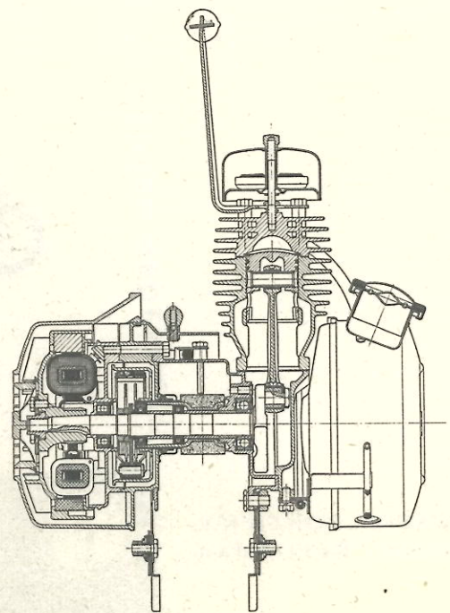
Doorsnede van de Solexmotor
